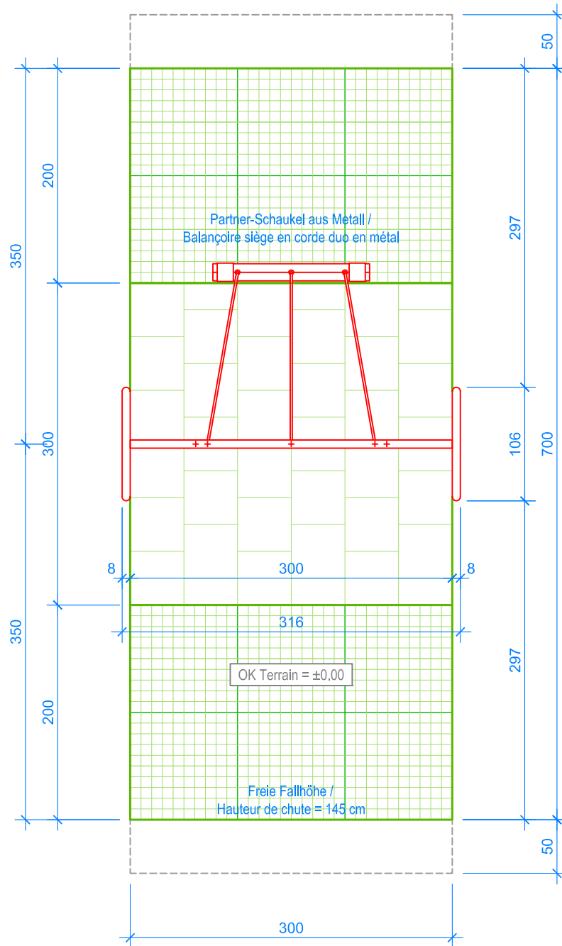
GRUNDRISS / PLAN 1:50
