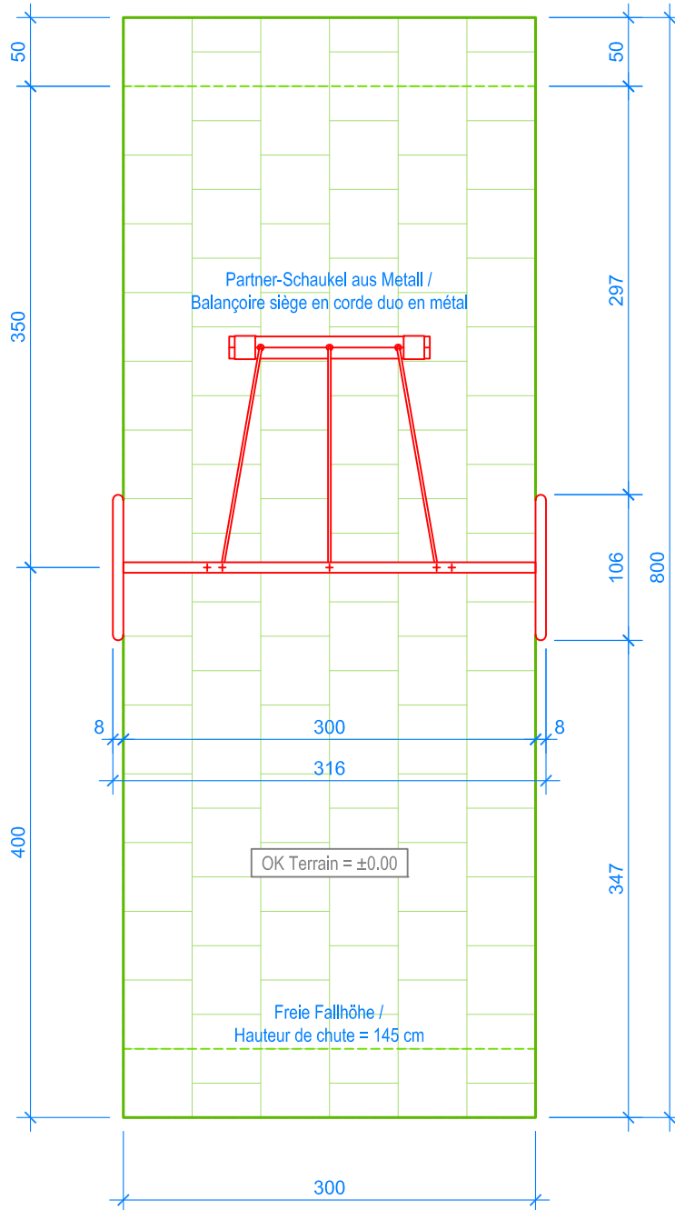
GRUNDRISS / PLAN 1:50
