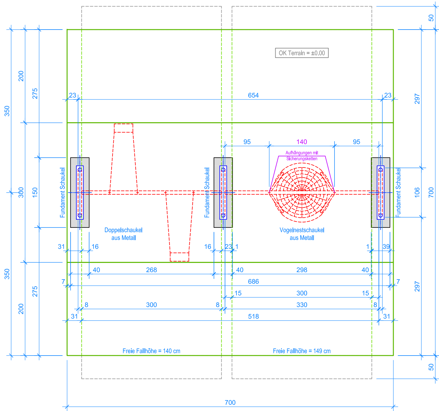
GRUNDRISS 1:50
