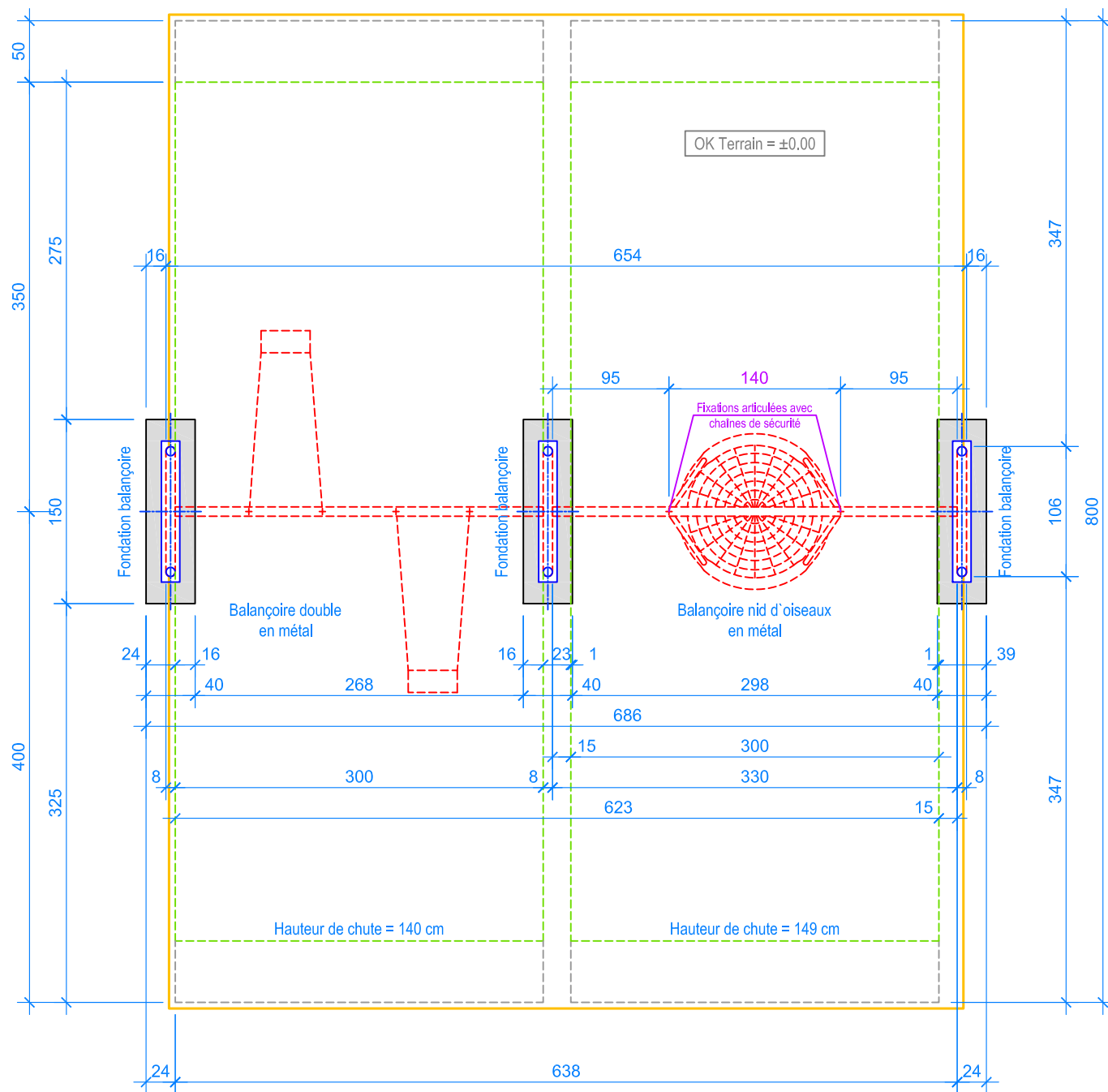
PLAN 1:50
