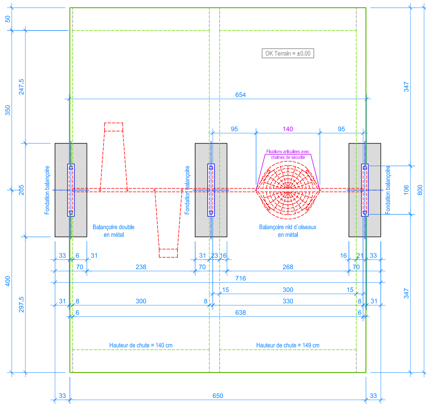
PLAN 1:50
