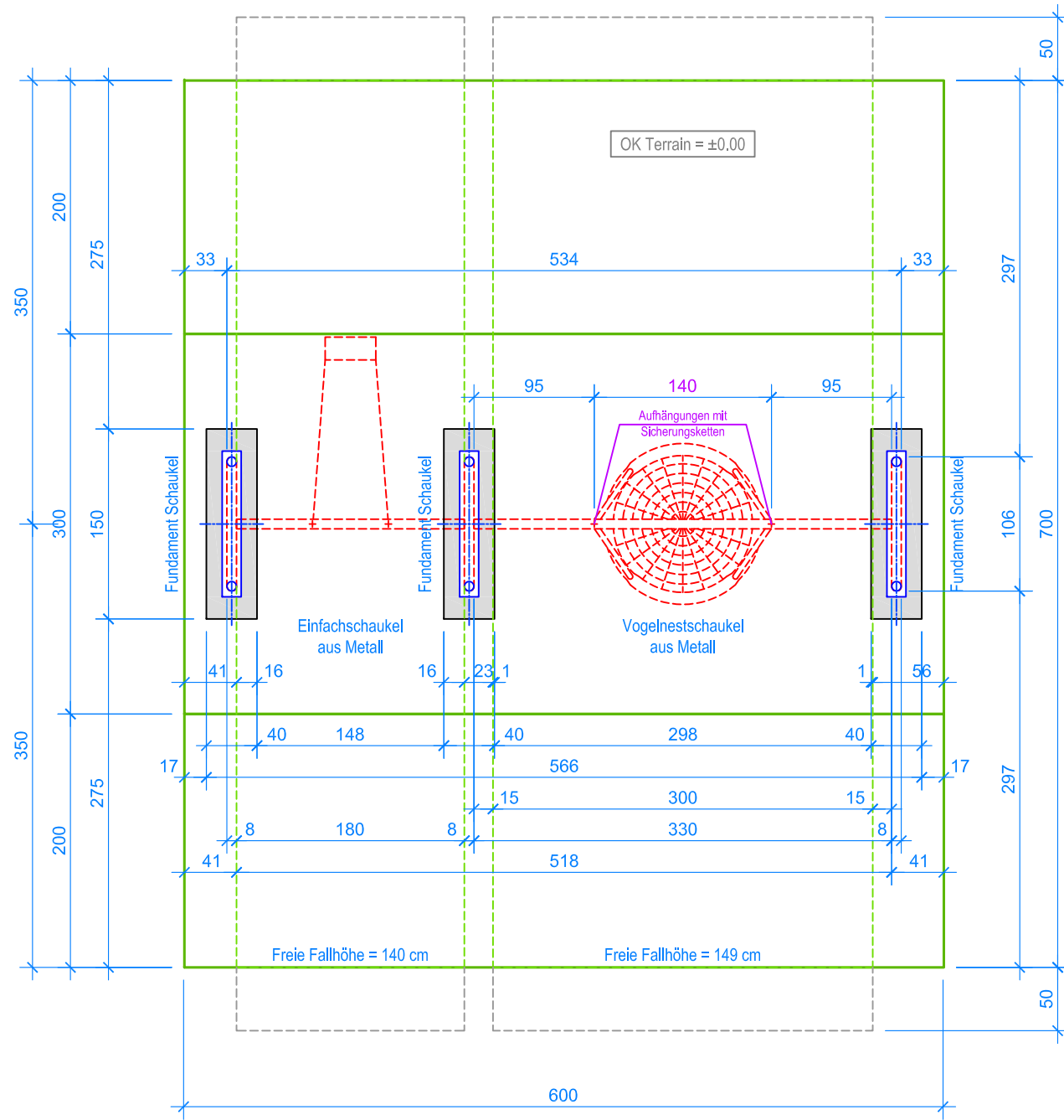
GRUNDRISS 1:50
