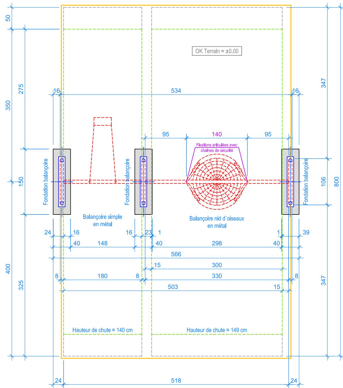
PLAN 1:50
