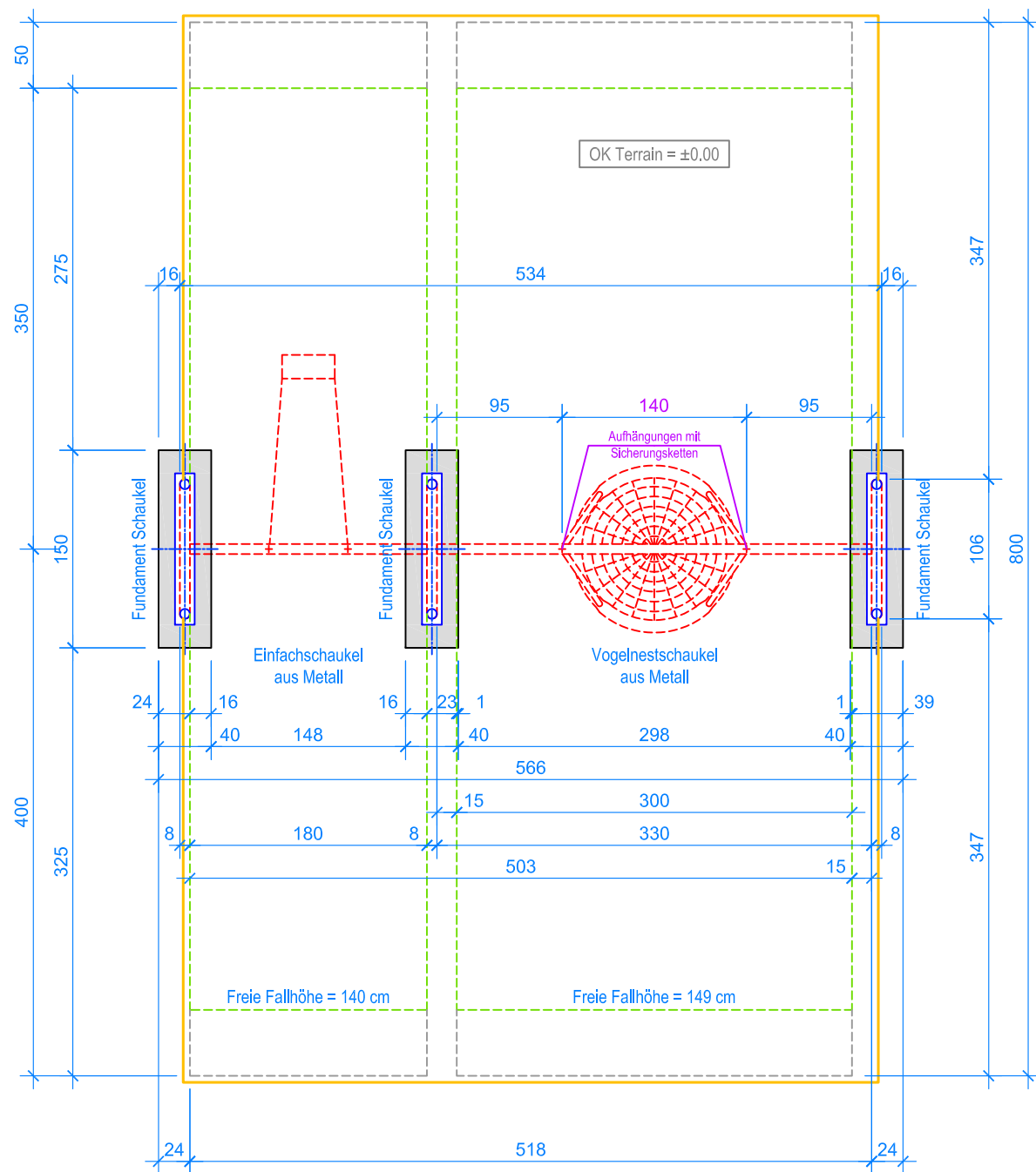
GRUNDRISS 1:50
