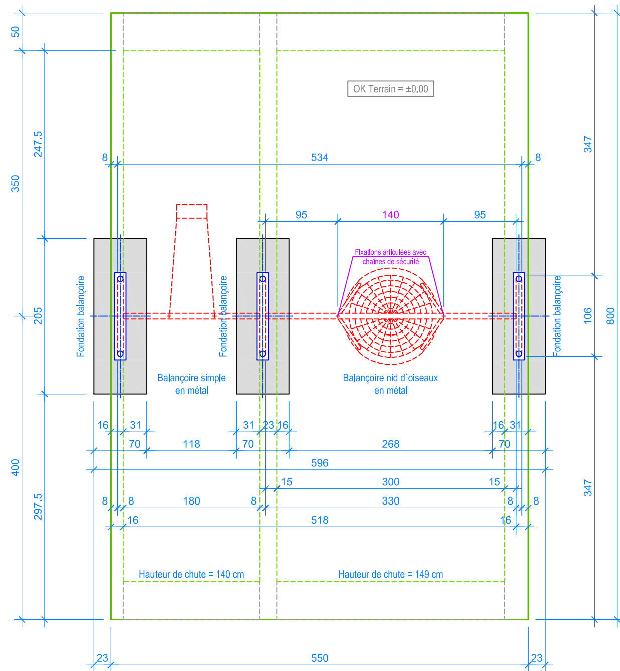
PLAN 1:50
