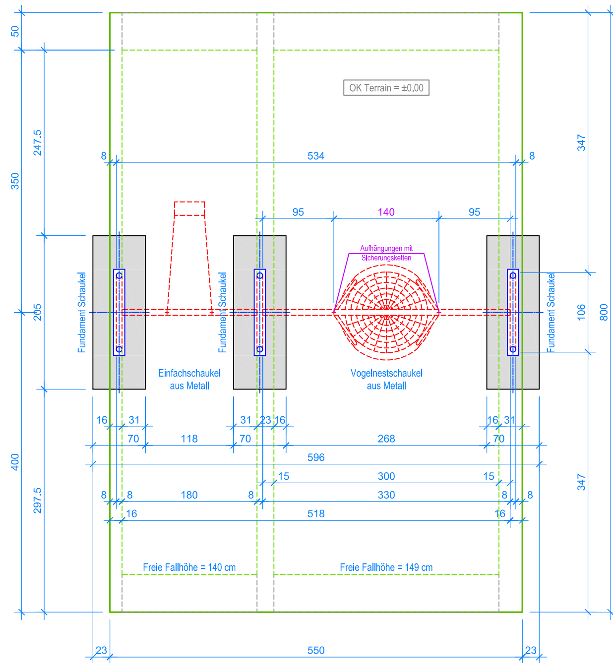
GRUNDRISS 1:50
