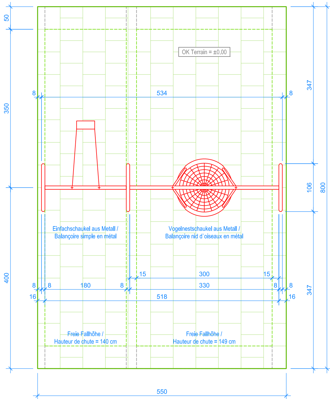
GRUNDRISS / PLAN 1:50
