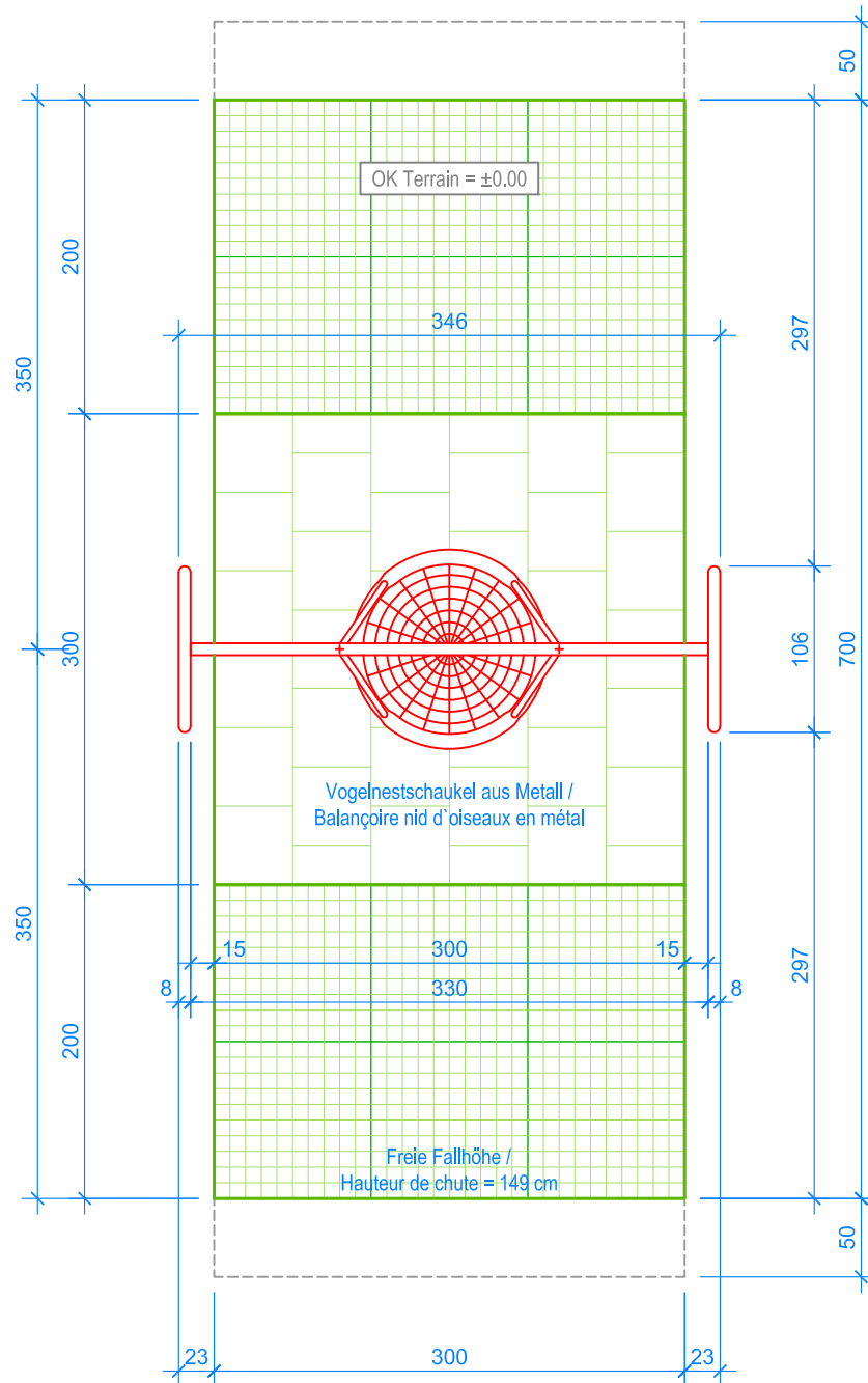
GRUNDRISS / PLAN 1:50
