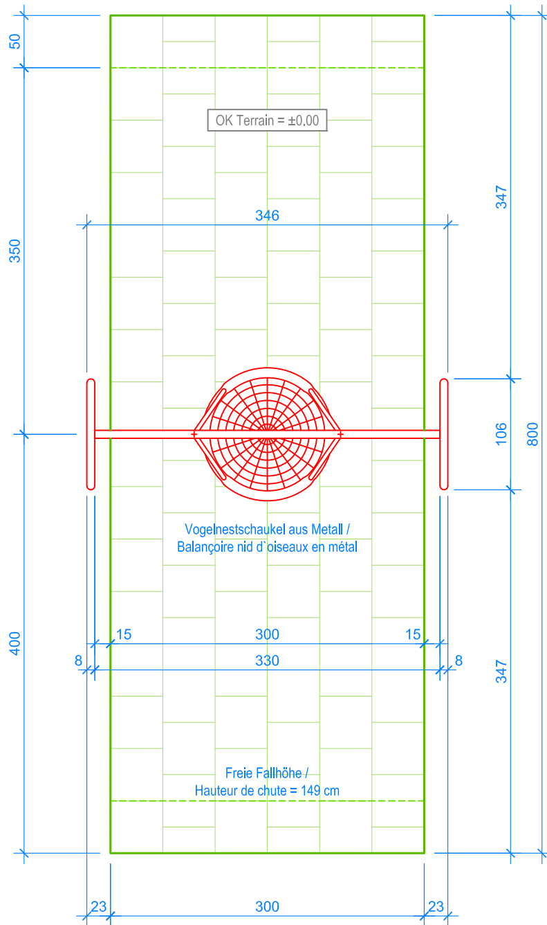
GRUNDRISS / PLAN 1:50
