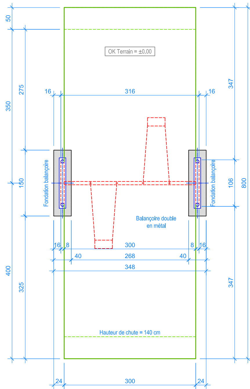
PLAN 1:50
