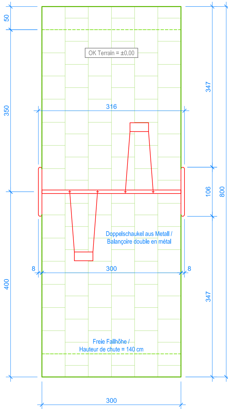
GRUNDRISS / PLAN 1:50
