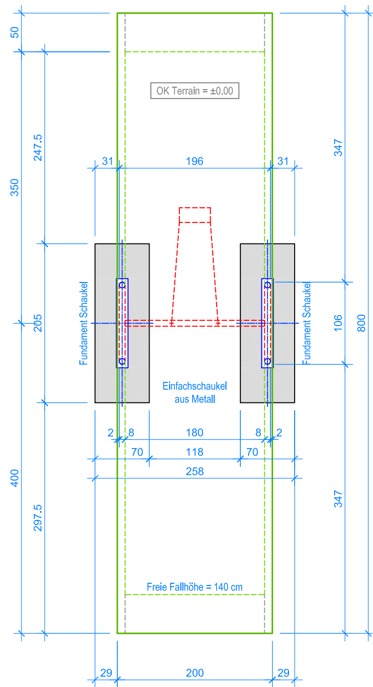
GRUNDRISS 1:50
