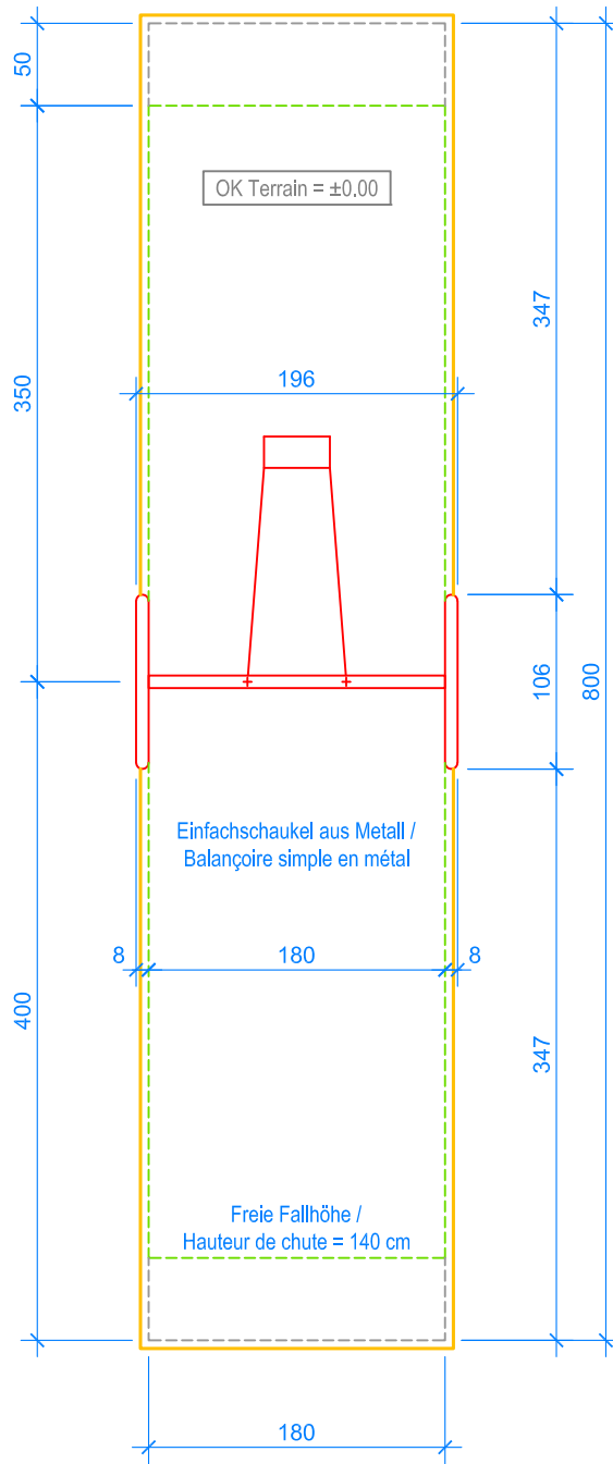
GRUNDRISS / PLAN 1:50
