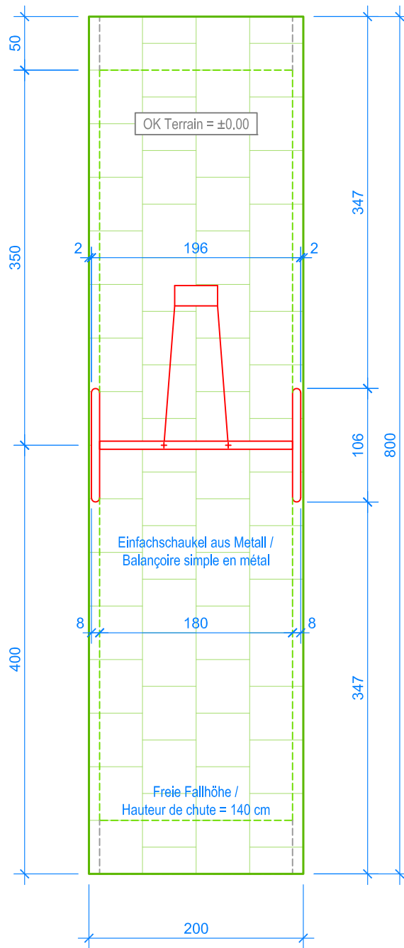
GRUNDRISS / PLAN 1:50
