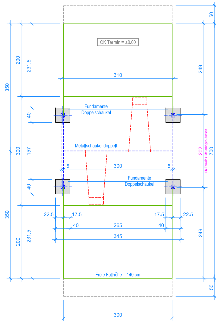
GRUNDRISS 1:50
