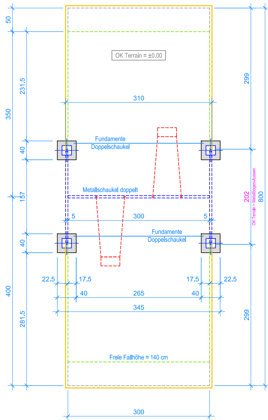
GRUNDRISS 1:50
