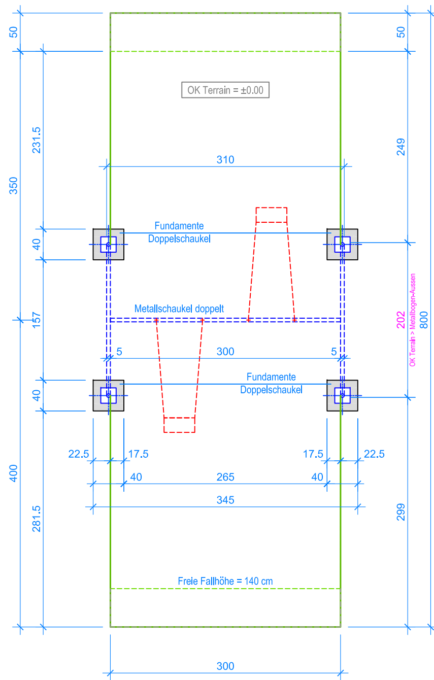
GRUNDRISS 1:50
