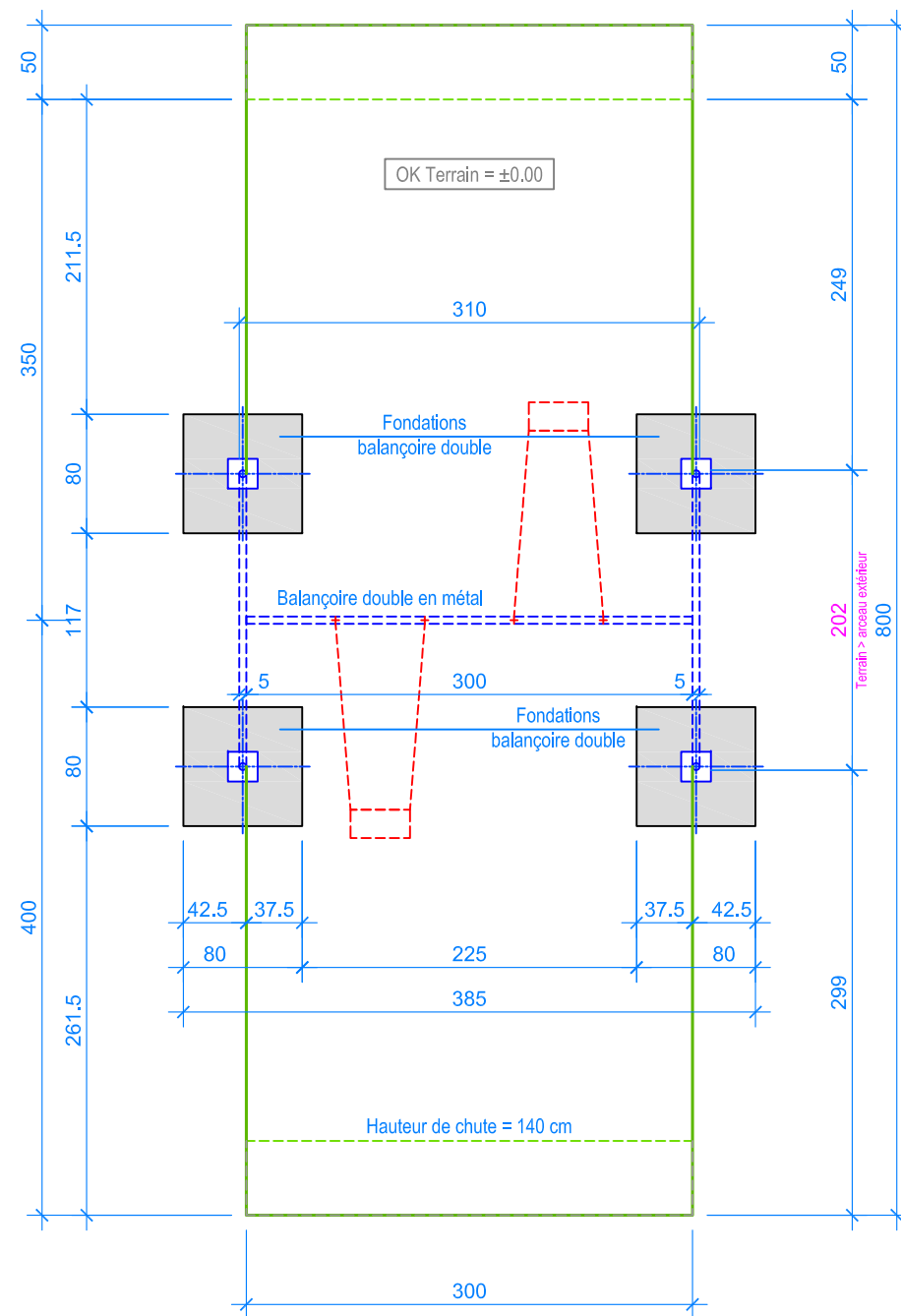
PLAN 1:50
