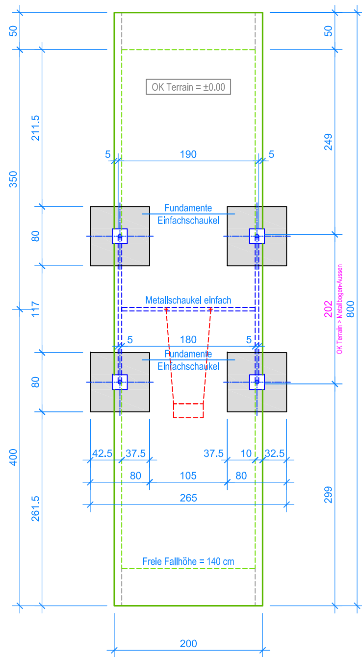
GRUNDRISS 1:50
