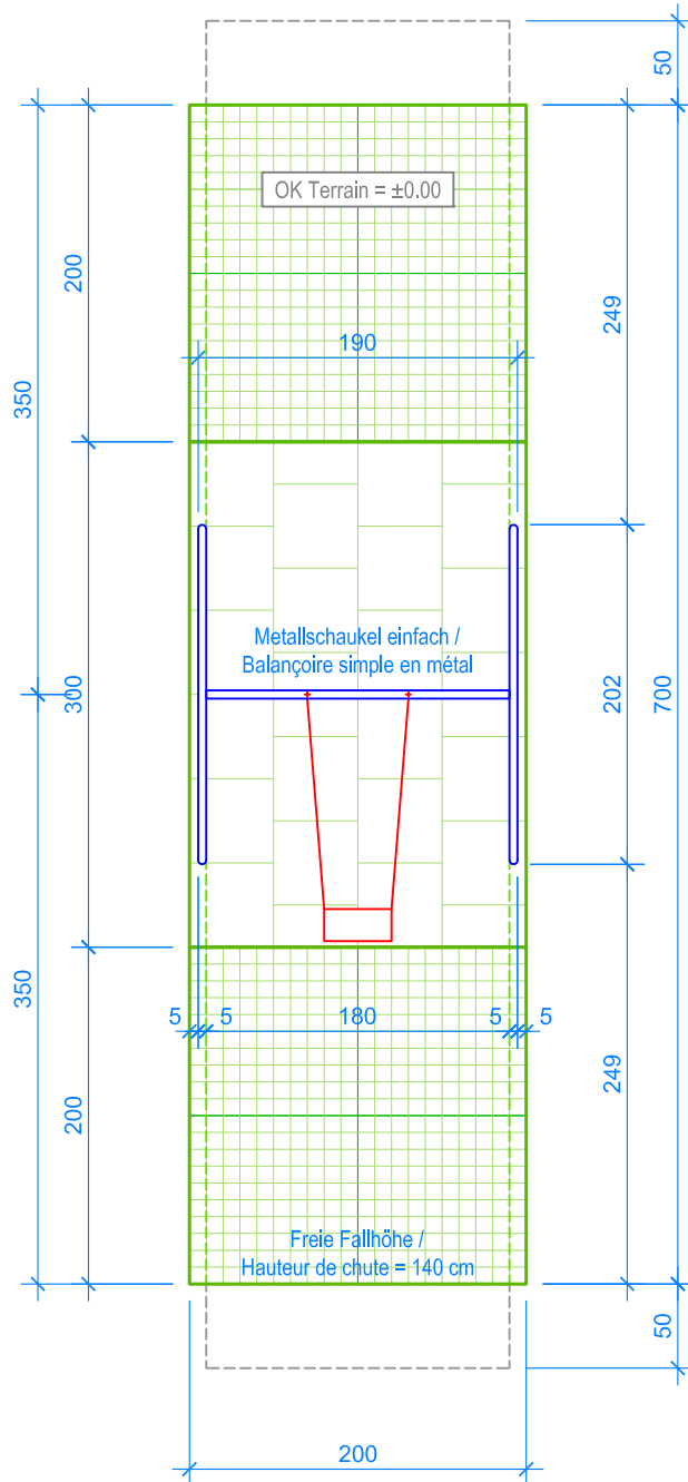
GRUNDRISS / PLAN 1:50
