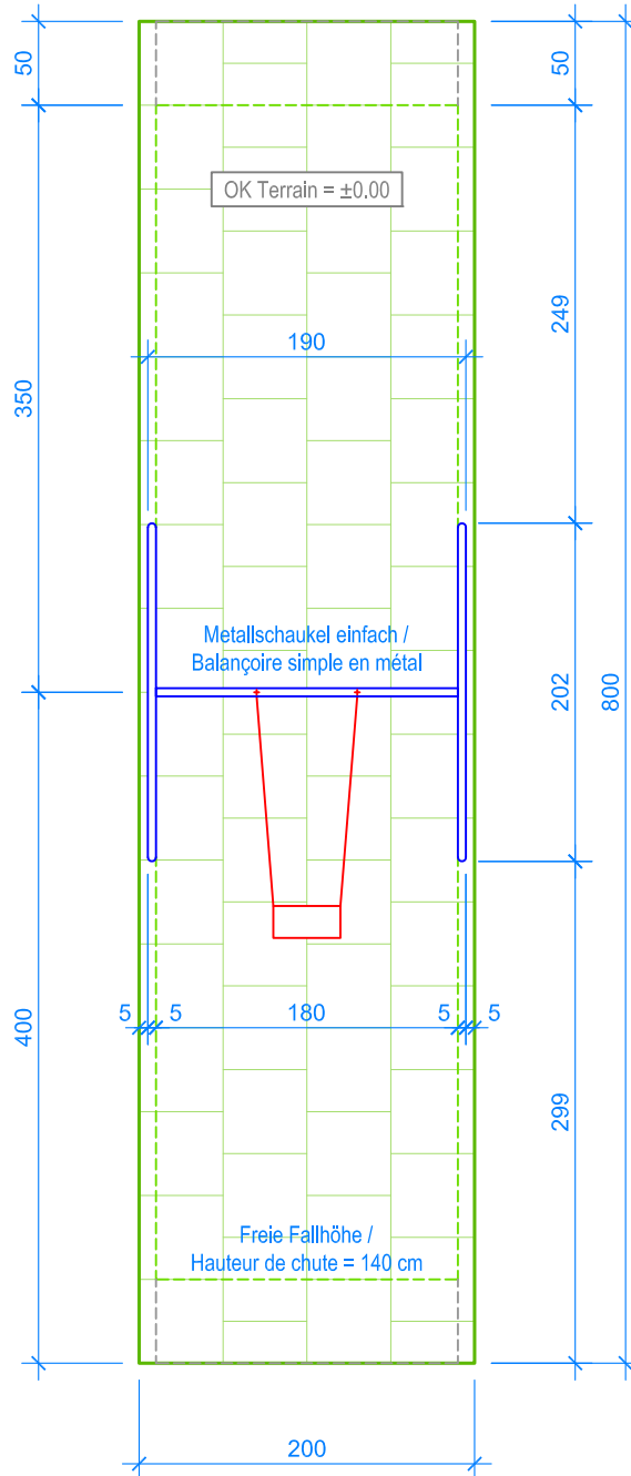
GRUNDRISS / PLAN 1:50
