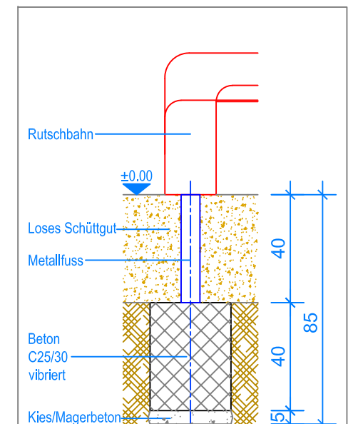
SCHNITT 1:20 FUNDAMENT PFOSTEN
