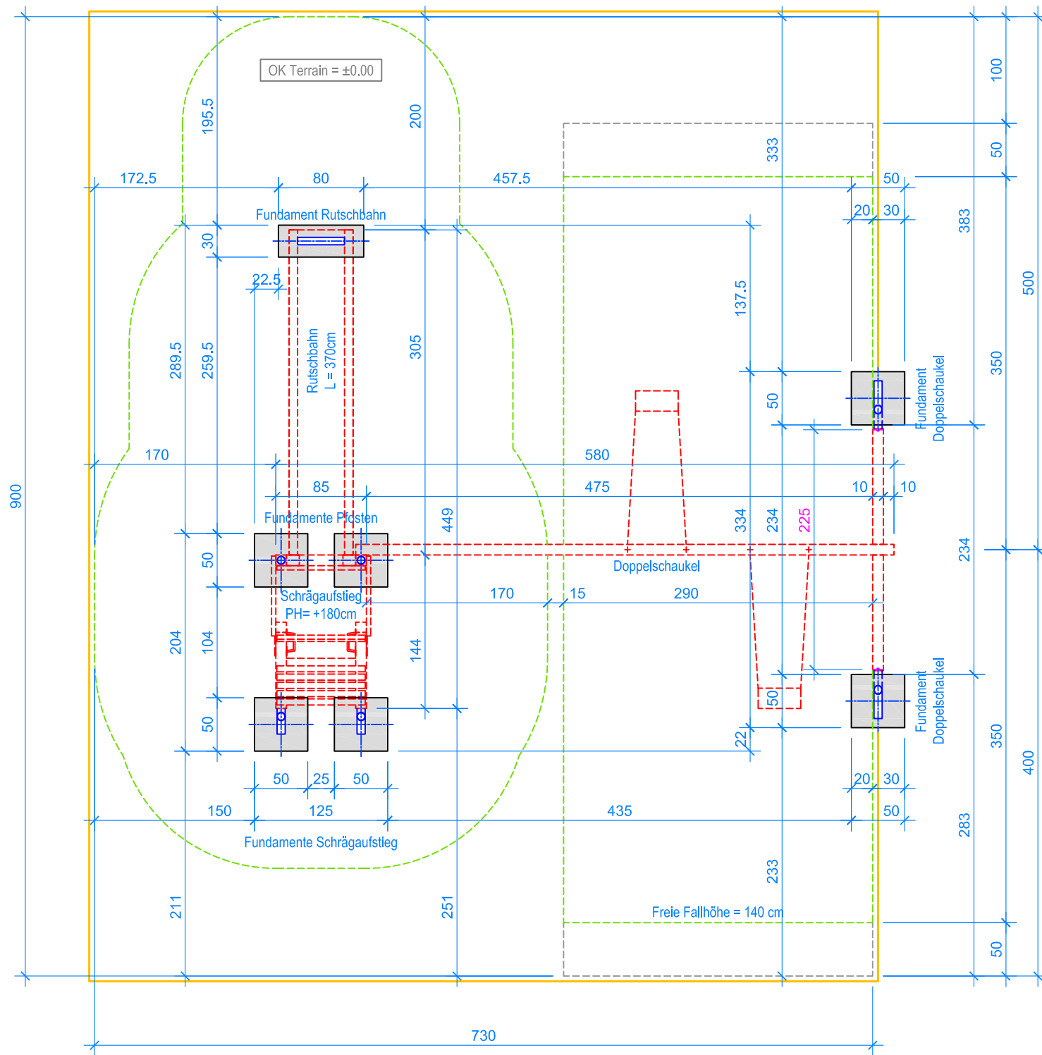
GRUNDRISS 1:50
