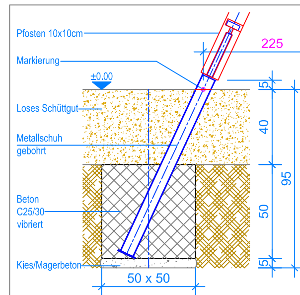
SCHNITT 1:20 FUNDAMENT DOPPELSCHAUKEL
