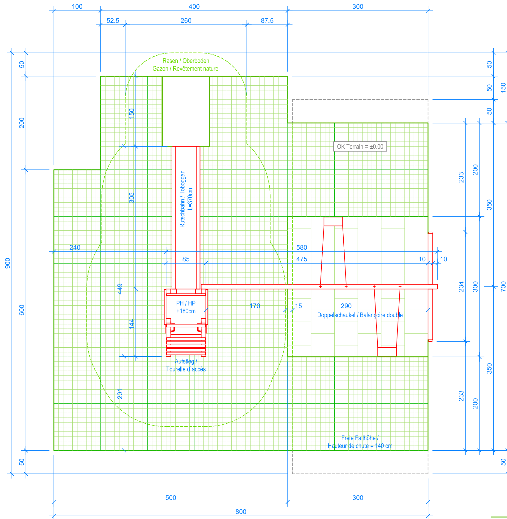
GRUNDRISS / PLAN 1:50
