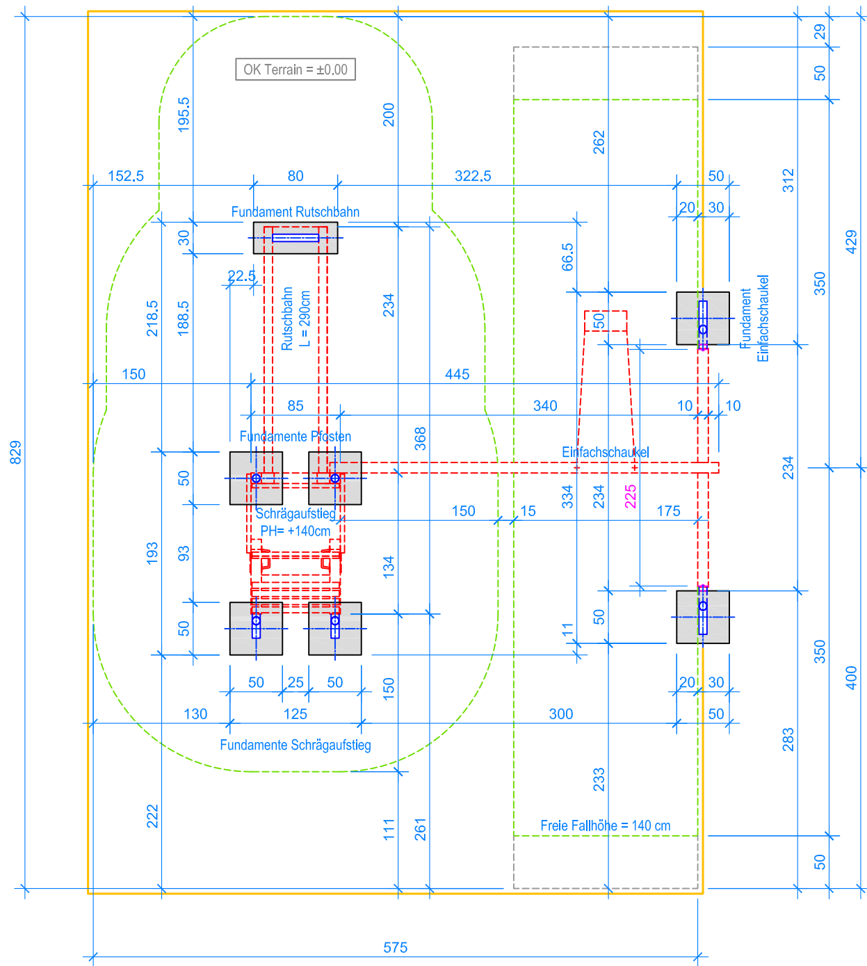
GRUNDRISS 1:50
