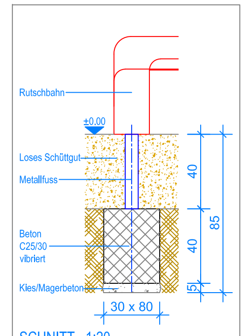
SCHNITT 1:20 FUNDAMENT RUTSCHBAHN
