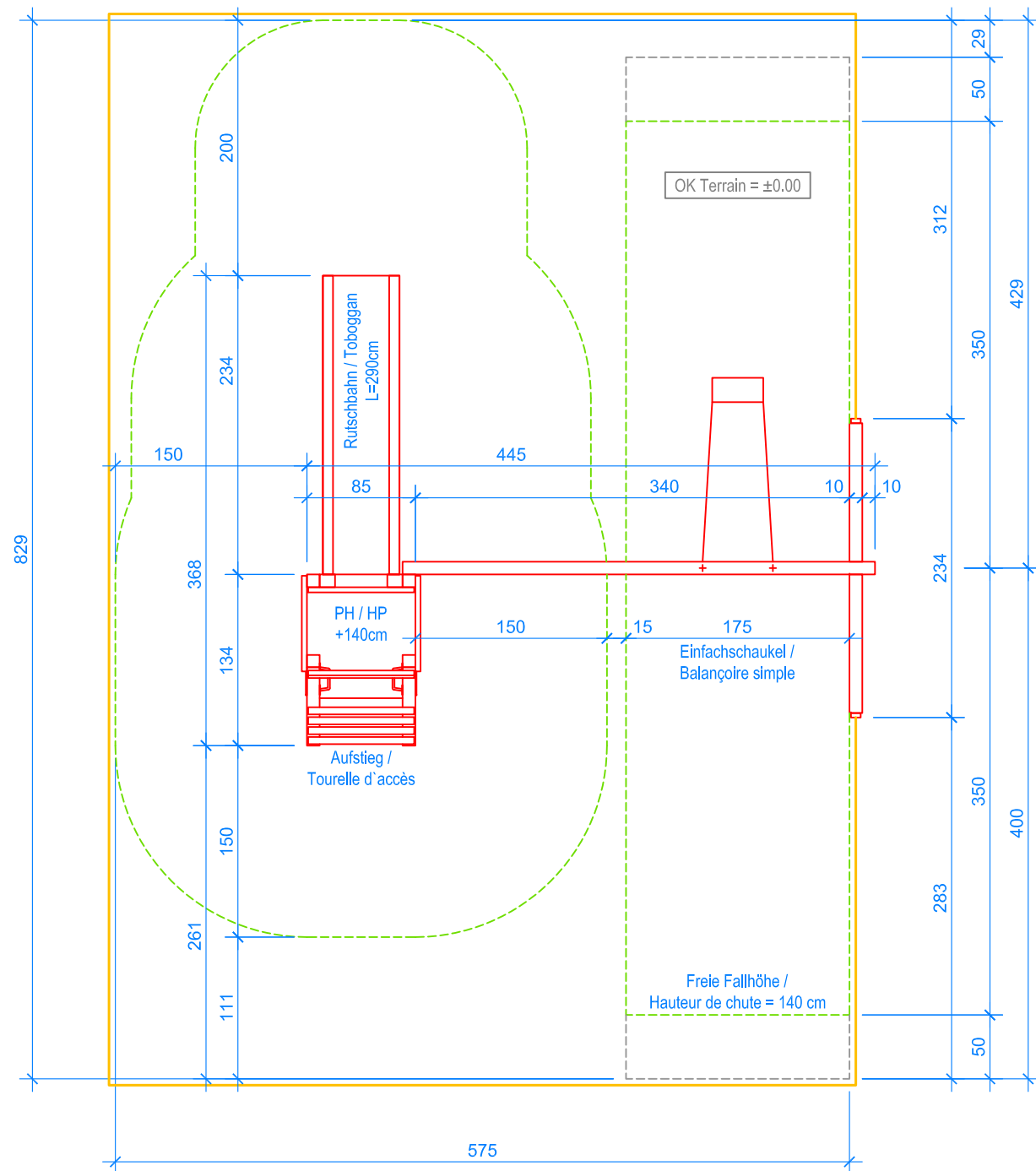
GRUNDRISS / PLAN 1:50
