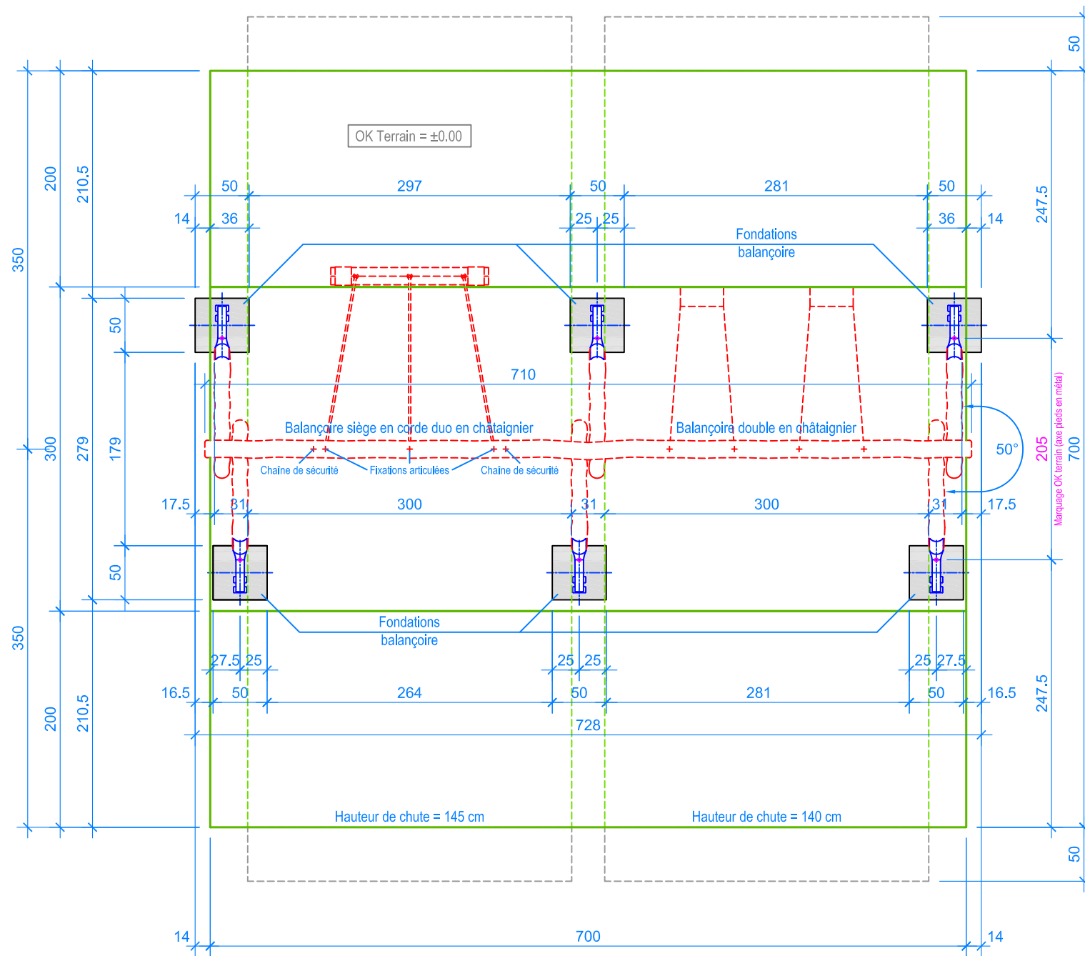
PLAN 1:50
