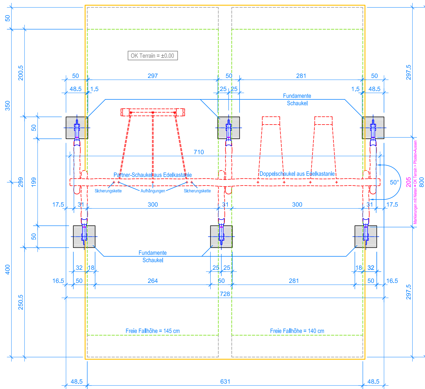
GRUNDRISS 1:50
