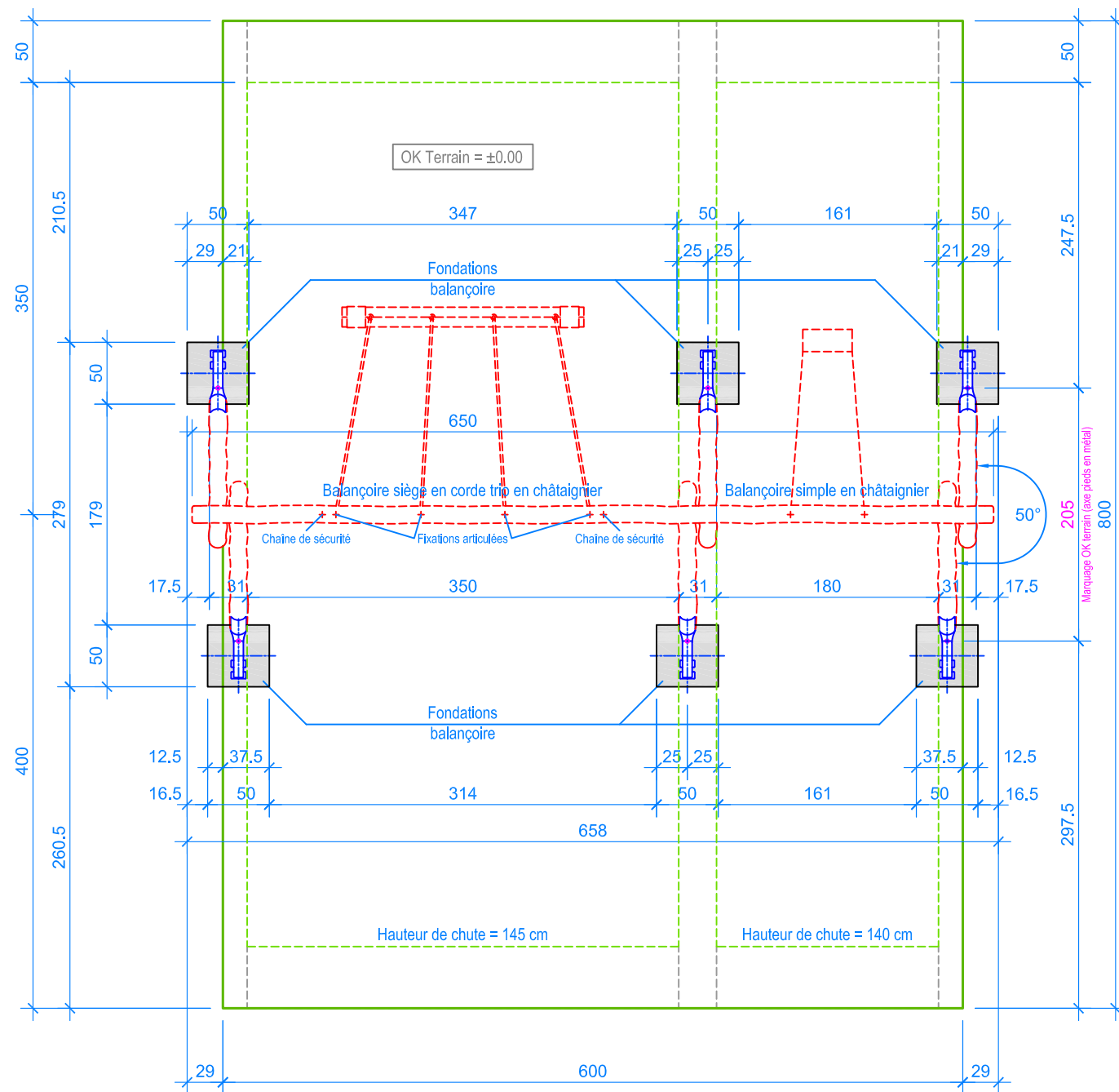
PLAN 1:50
