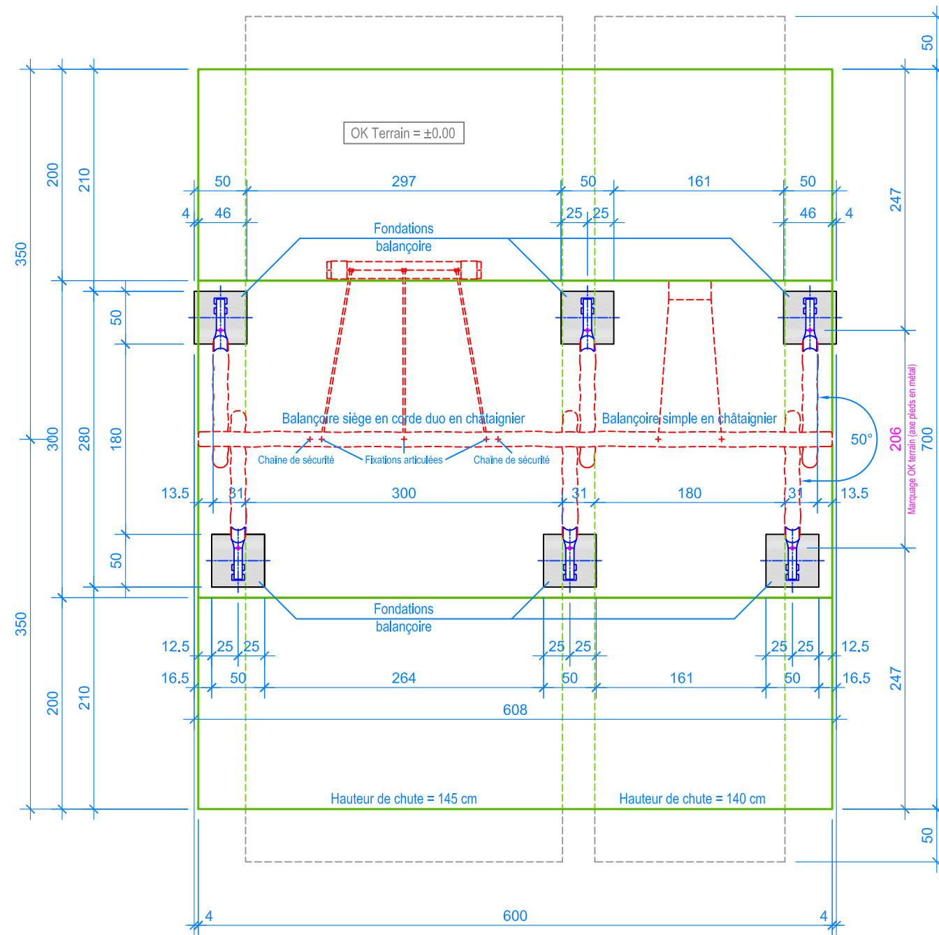
PLAN 1:50
