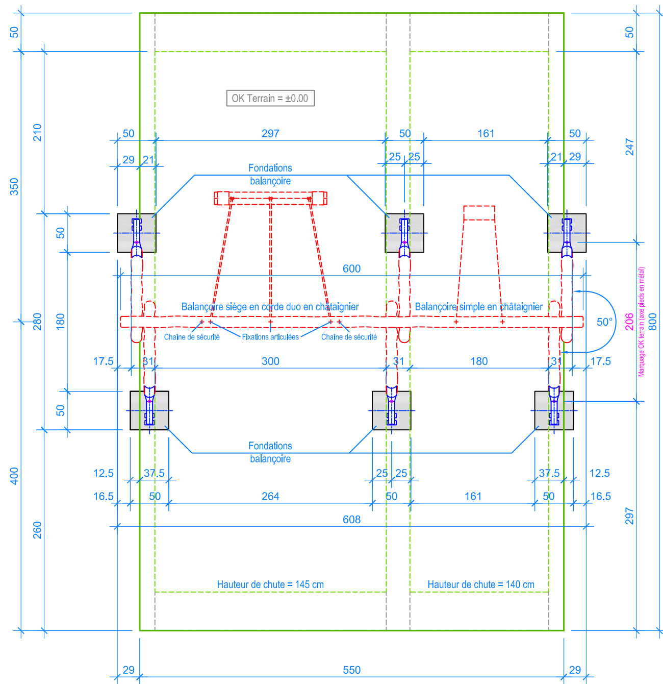
PLAN 1:50
