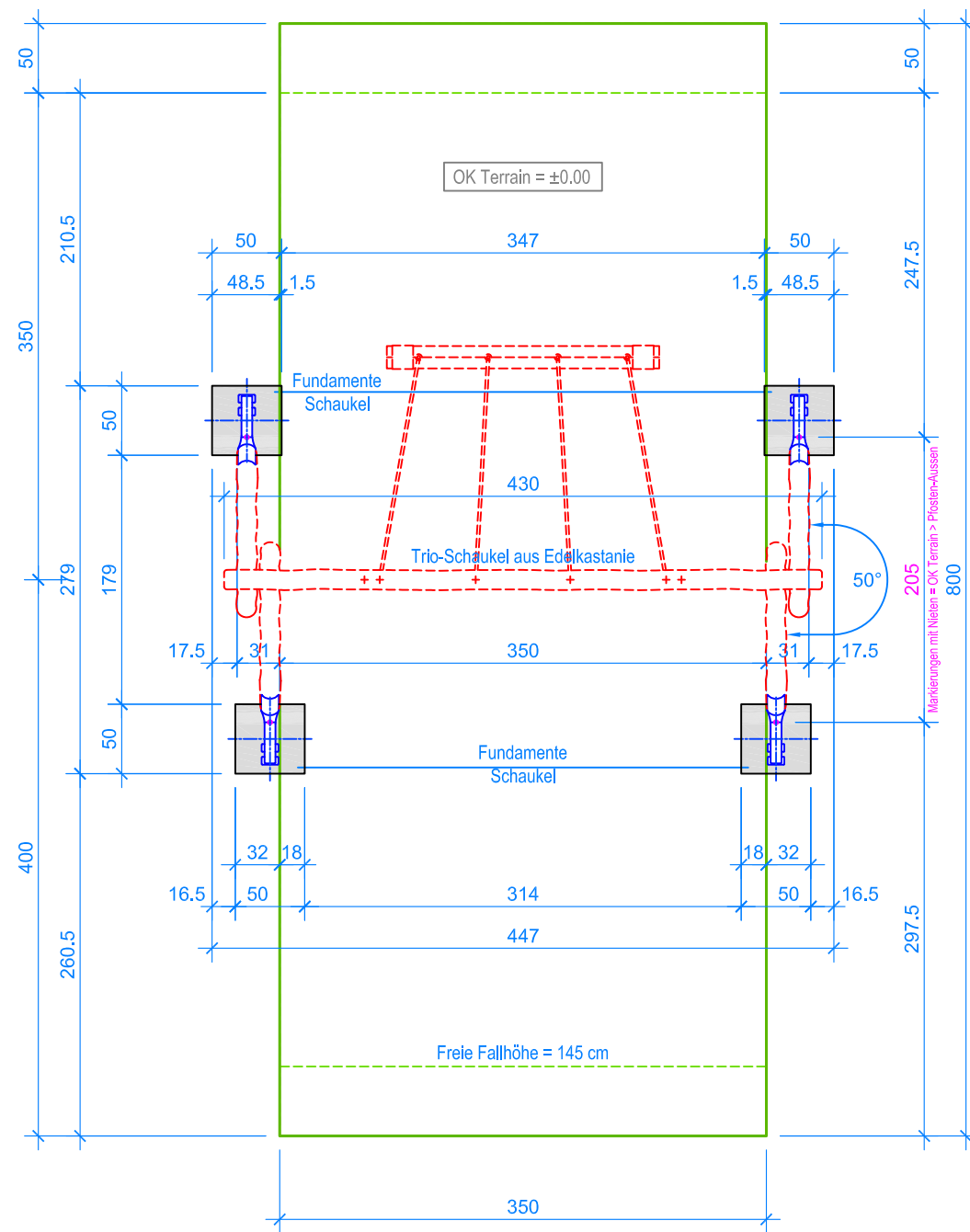
GRUNDRISS 1:50
