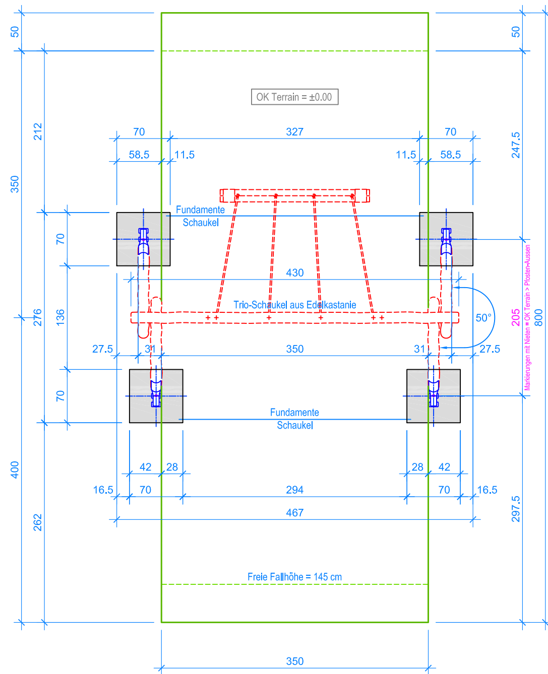
GRUNDRISS 1:50
