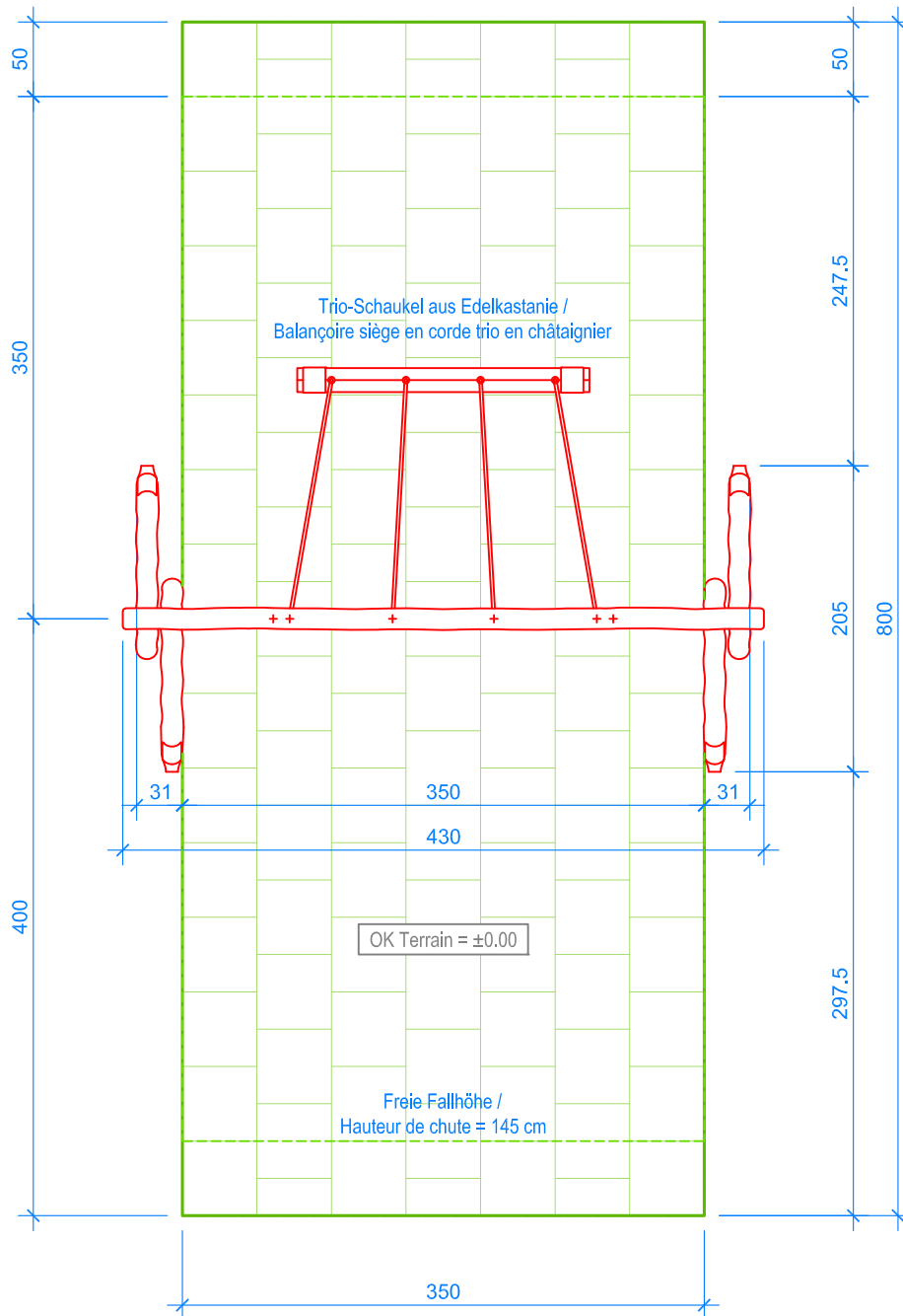
GRUNDRISS / PLAN 1:50
