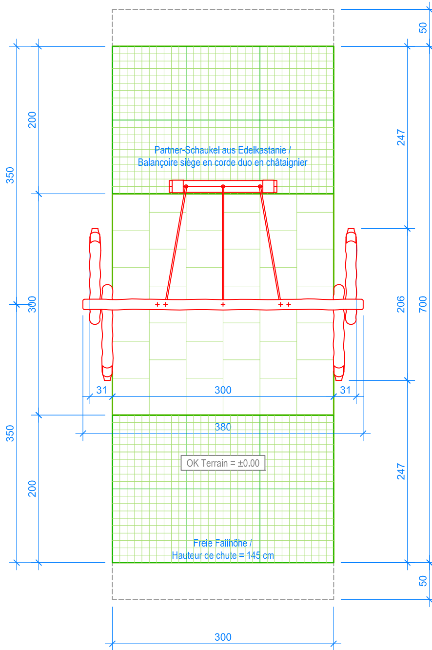
GRUNDRISS / PLAN 1:50
