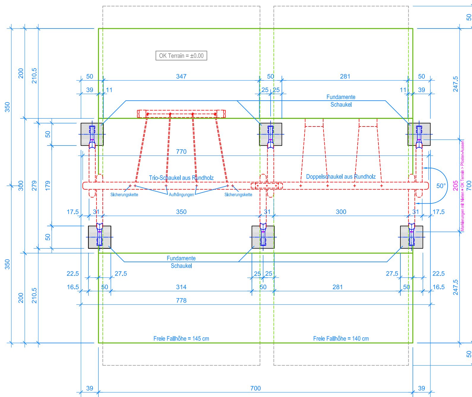
GRUNDRISS 1:50
