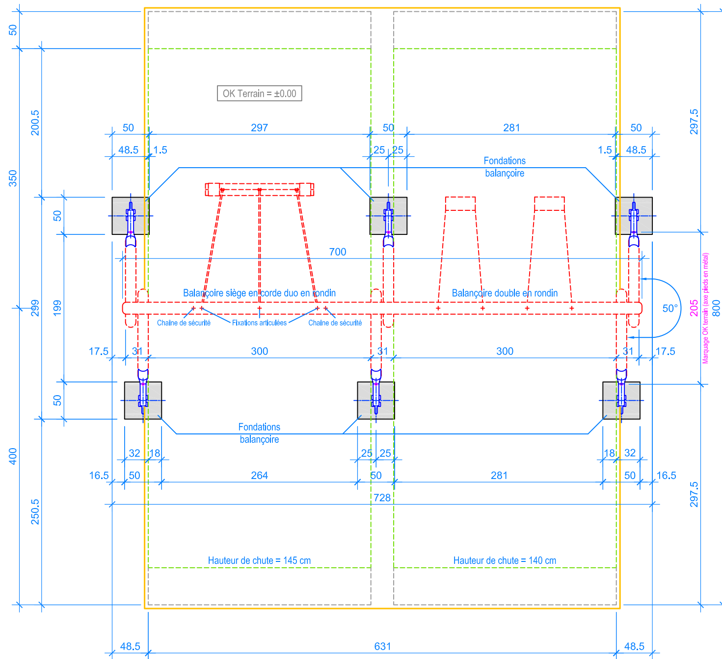
PLAN 1:50
