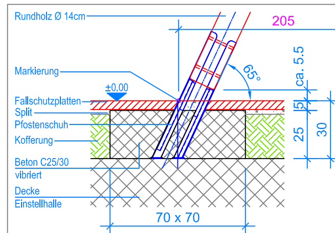
SCHNITT 1:20 FUNDAMENT SCHAUKEL
