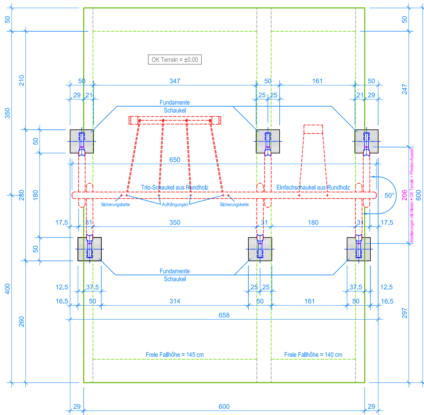
GRUNDRISS 1:50
