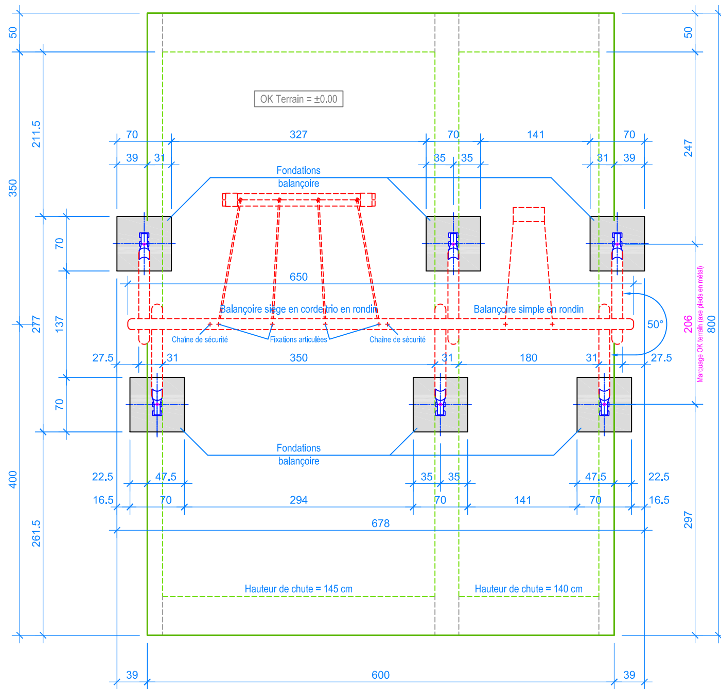
PLAN 1:50
