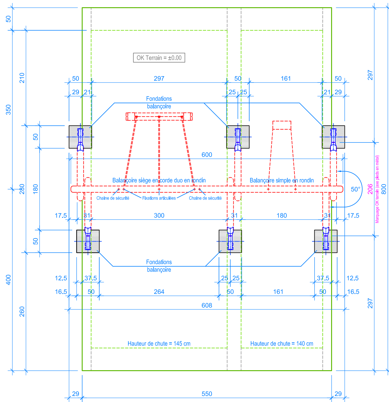
PLAN 1:50
