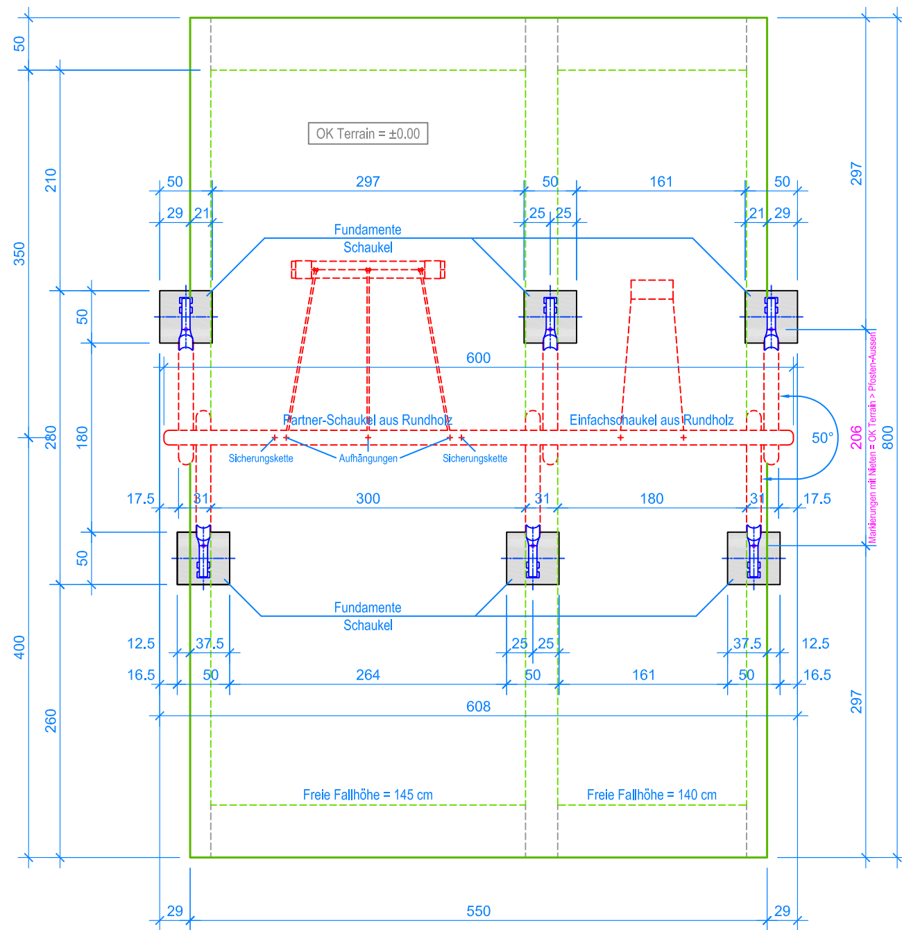
GRUNDRISS 1:50
