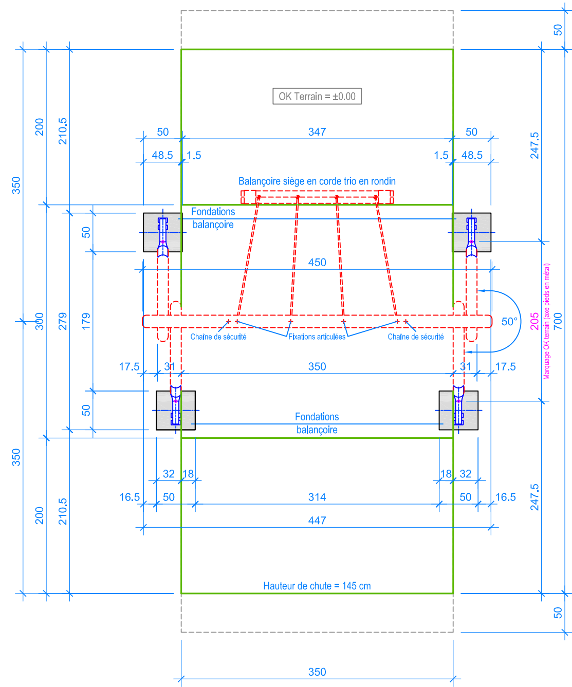
PLAN 1:50
