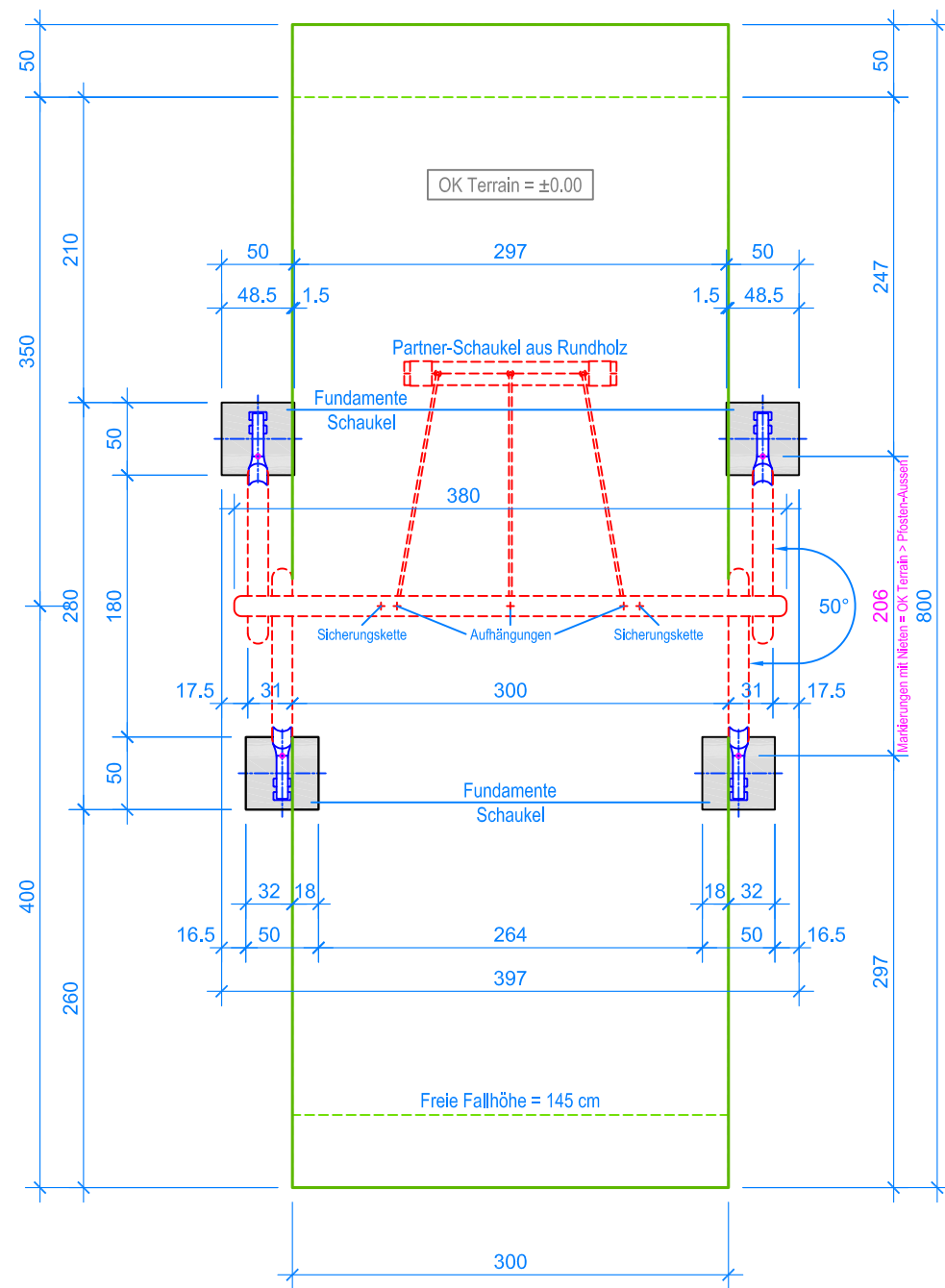
GRUNDRISS 1:50
