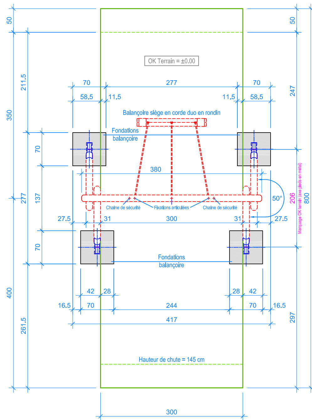
PLAN 1:50
