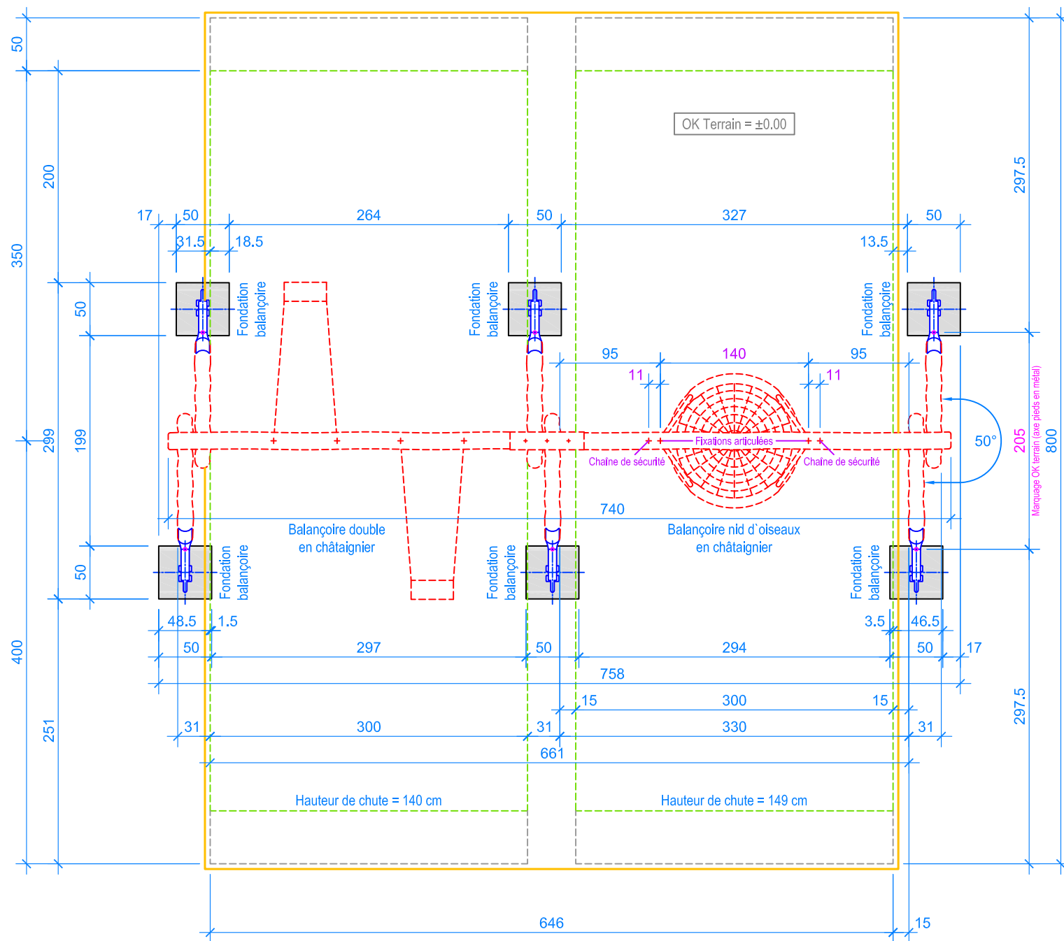
PLAN 1:50
