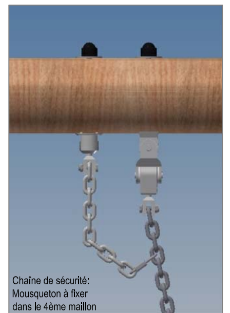
Détail A
