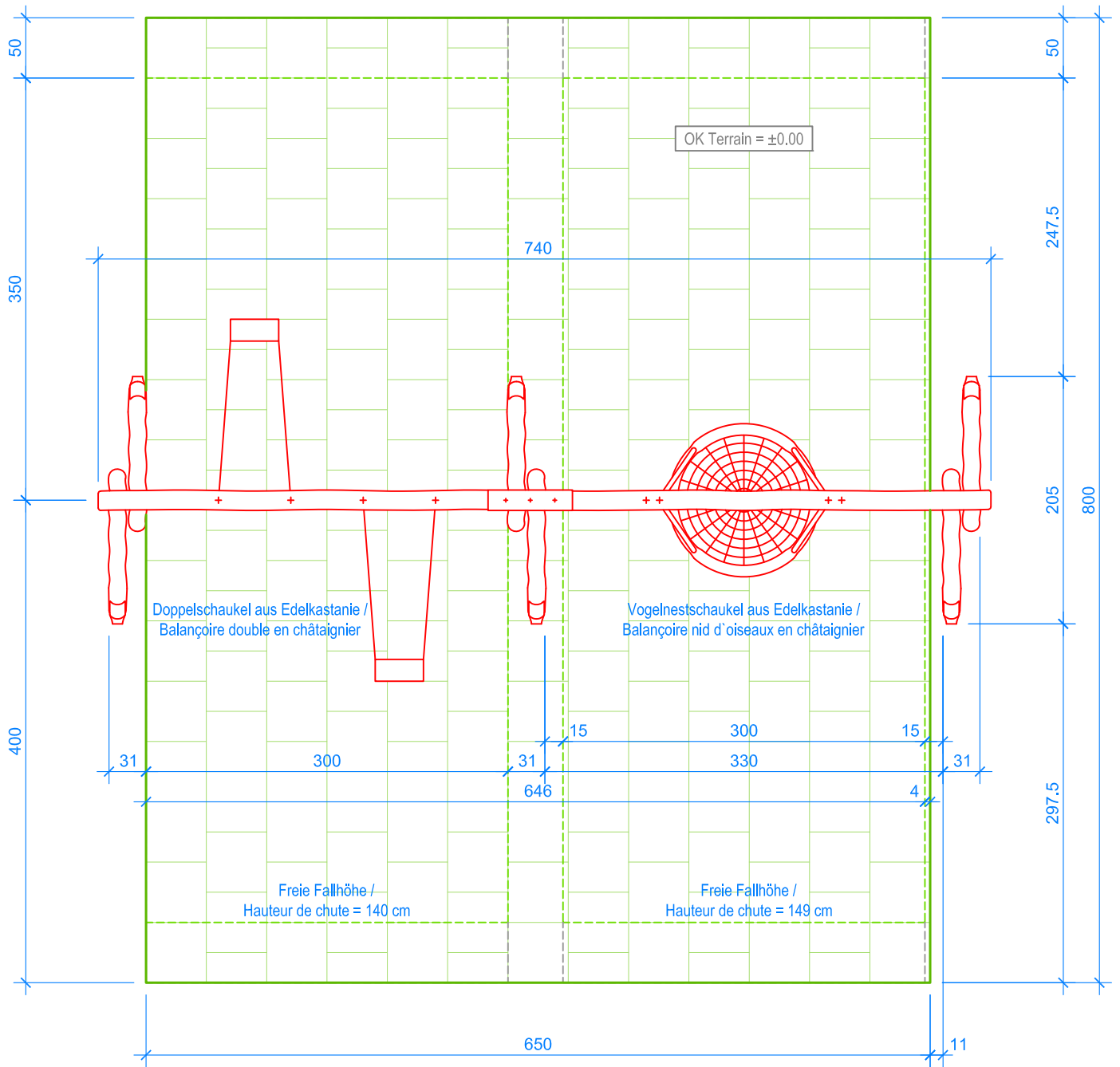
GRUNDRISS / PLAN 1:50
